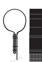
3" Pocket (max pipe OD = 1.029")
